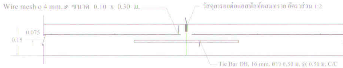
ดูแบบขยาย ② รอยต่อตามยาว
