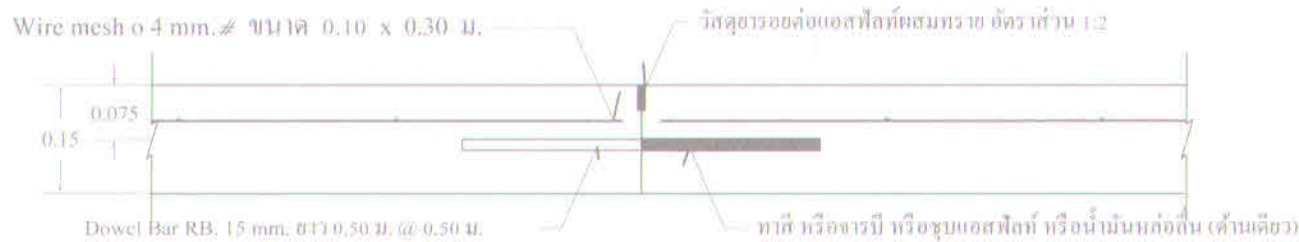
ดูแบบขยาย ③ รอยต่อหดตัวตามขวาง ทุกระยะไม่เกิน 10.00 ม.
