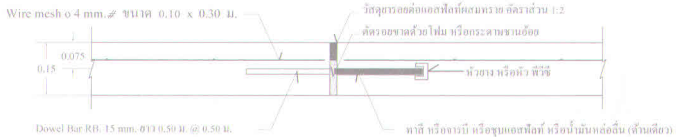
ดูแบบขยาย ① รอยต่อขยายตัวตามขวาง ทุกระยะ 50 ม. (คอนกรีตตัดขาด)
