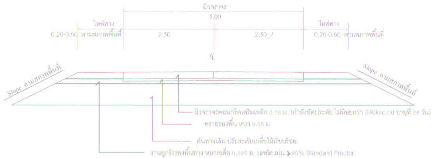
รูปตัดโครงสร้าง
